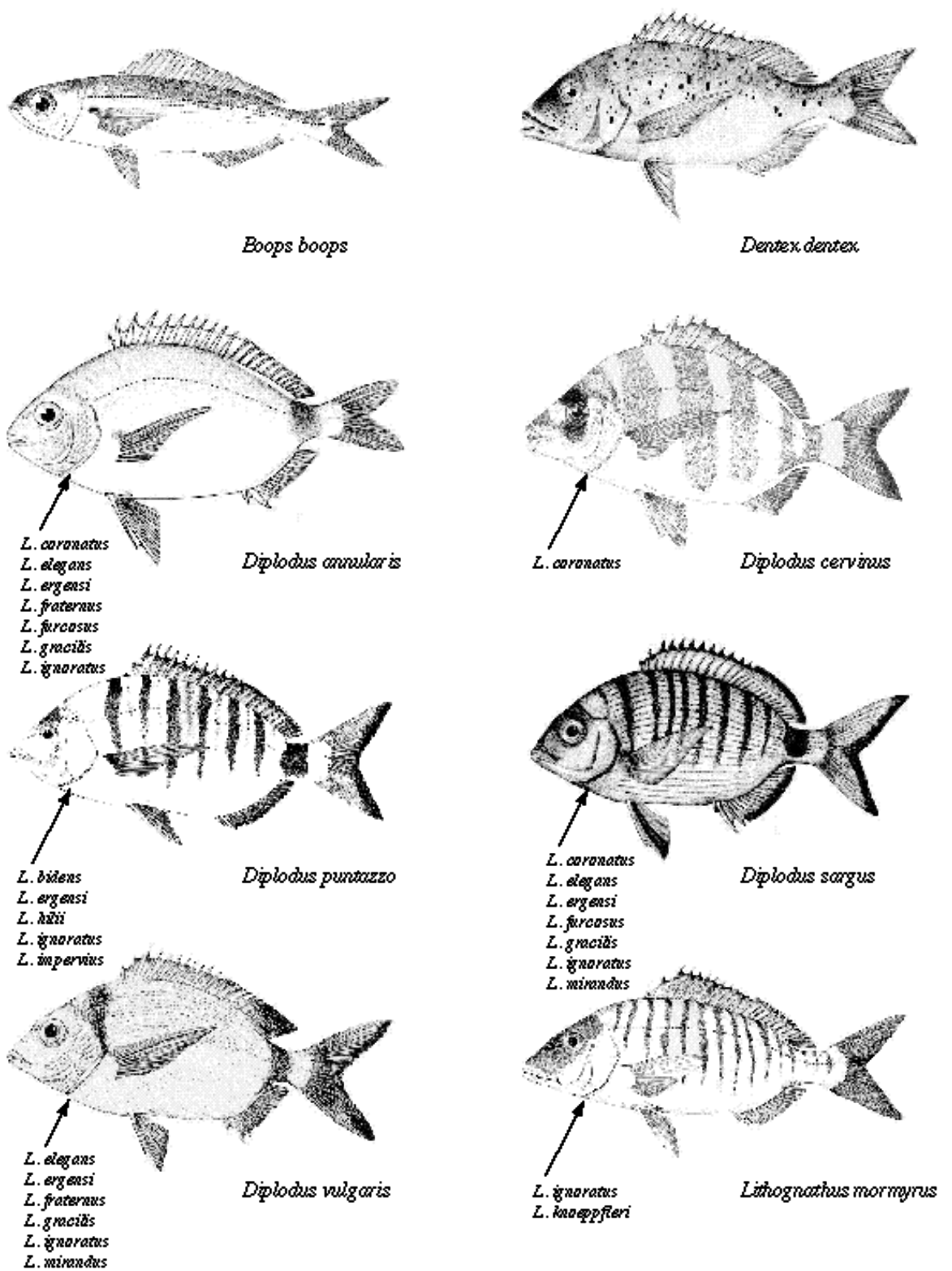
Figure II.3 : Espèces de Sparidae étudiées. Les espèces de Lamellodiscus qui s'y trouvent sont mentionnées.
