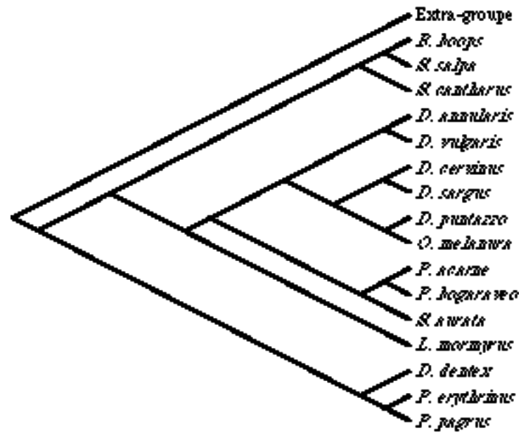
Figure IV.10 : Arbre phylogénétique des Sparidae obtenu par maximum de vraisemblance à partir des séquences 16S + cyt-b.
