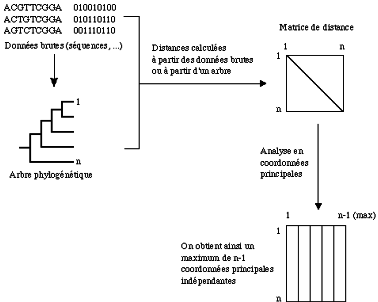
Figure II.7 : Transformation des relations phylogénétiques en coordonnées principales.
