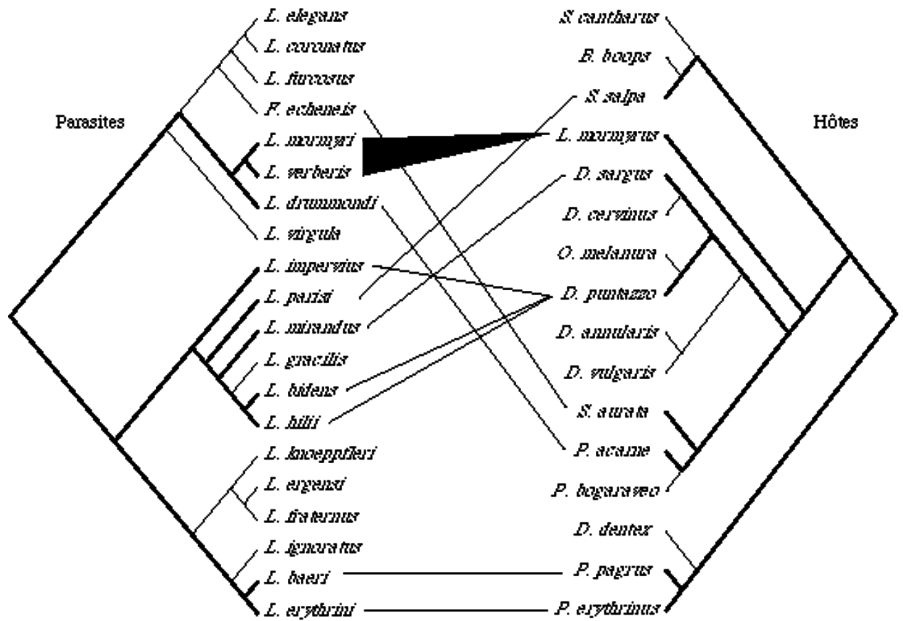
Figure IV.16 : Profil de coevolution hôte-parasite chez les espèces de Lamellodiscus spécialistes.
