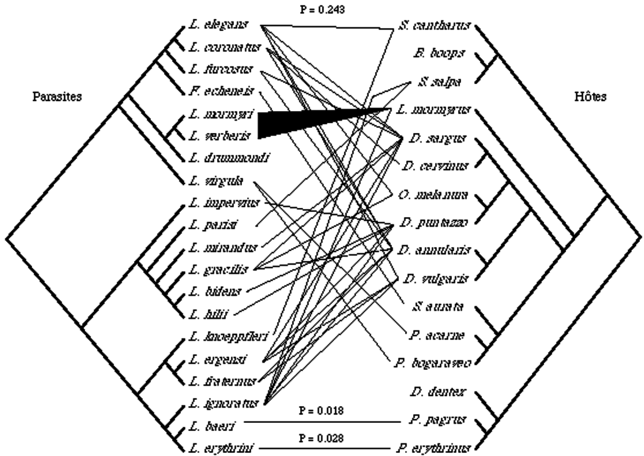
Figure IV.12 : Profil d'association coévolutive entre Sparidae et Lamellodiscus .
