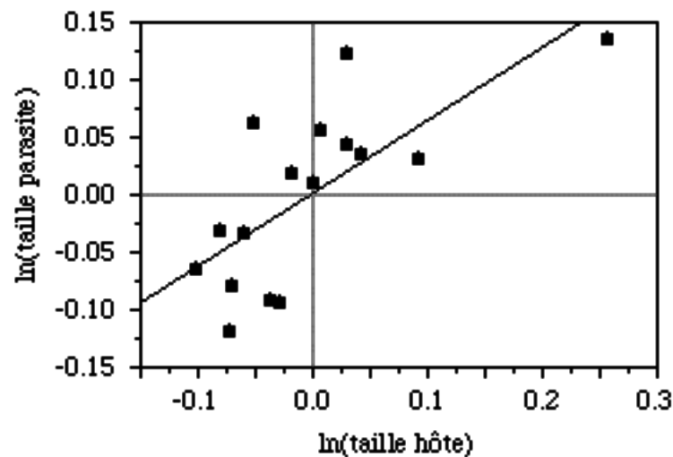
Figure IV.22 : Lien entre la taille des parasites et la taille de l'hôte chez les Lamellodiscus ( r = 0.719 , P = 0.004 ).
