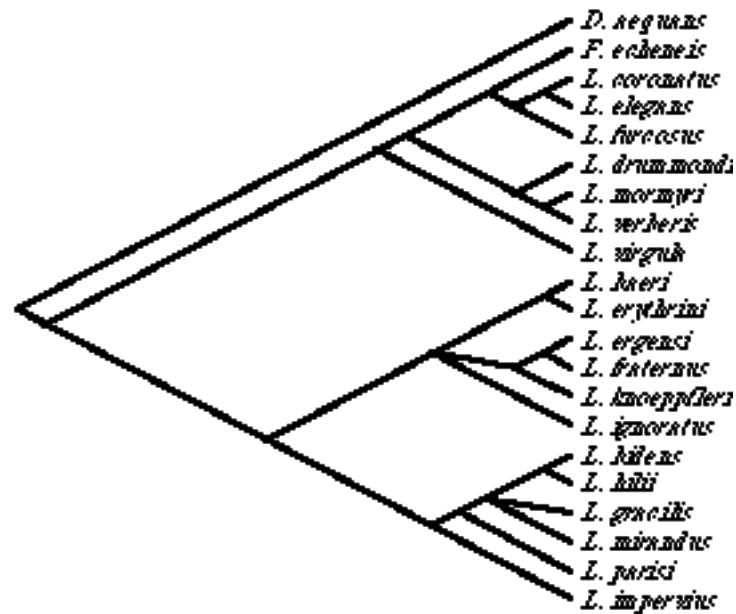
Figure IV.7 : Arbre phylogénétique des Lamellodiscus obtenu par maximum de vraisemblance.
