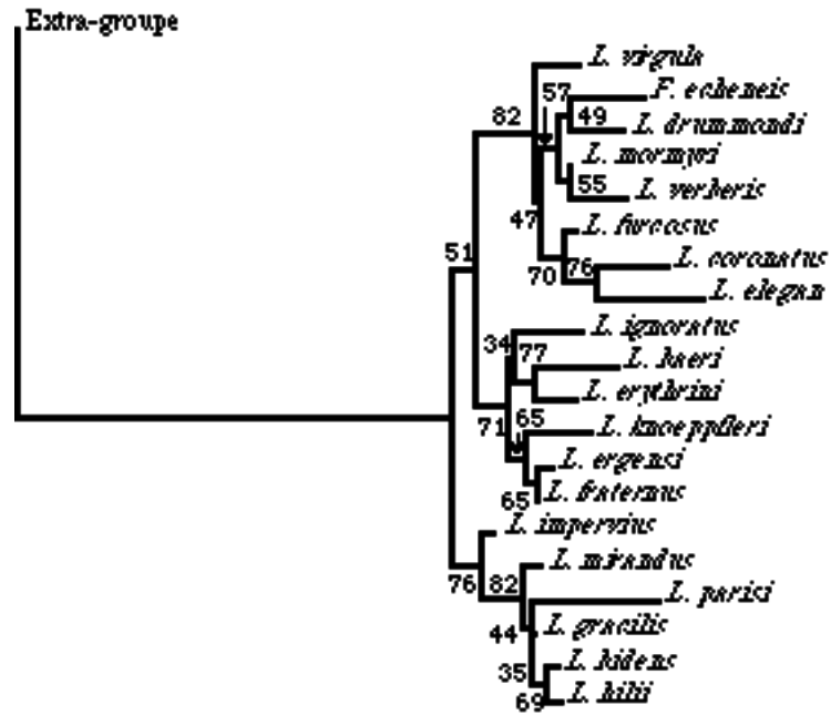
Figure IV.6 : Arbre phylogénétique des Lamellodiscus obtenus par "neighbour-joining". Les nombres sont les valeurs de bootstrap, en pourcentage (1000 répliqués).
