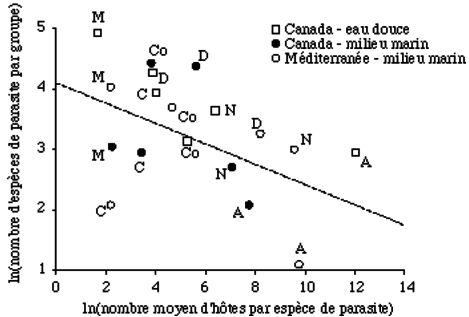
Figure IV.1: Lien entre la spécificité (nombre d'hôtes) et la diversification taxonomique (nombre d'espèces par groupe) pour les principaux groupes de parasites ( r = 0.510 , P = 0.027 ).
