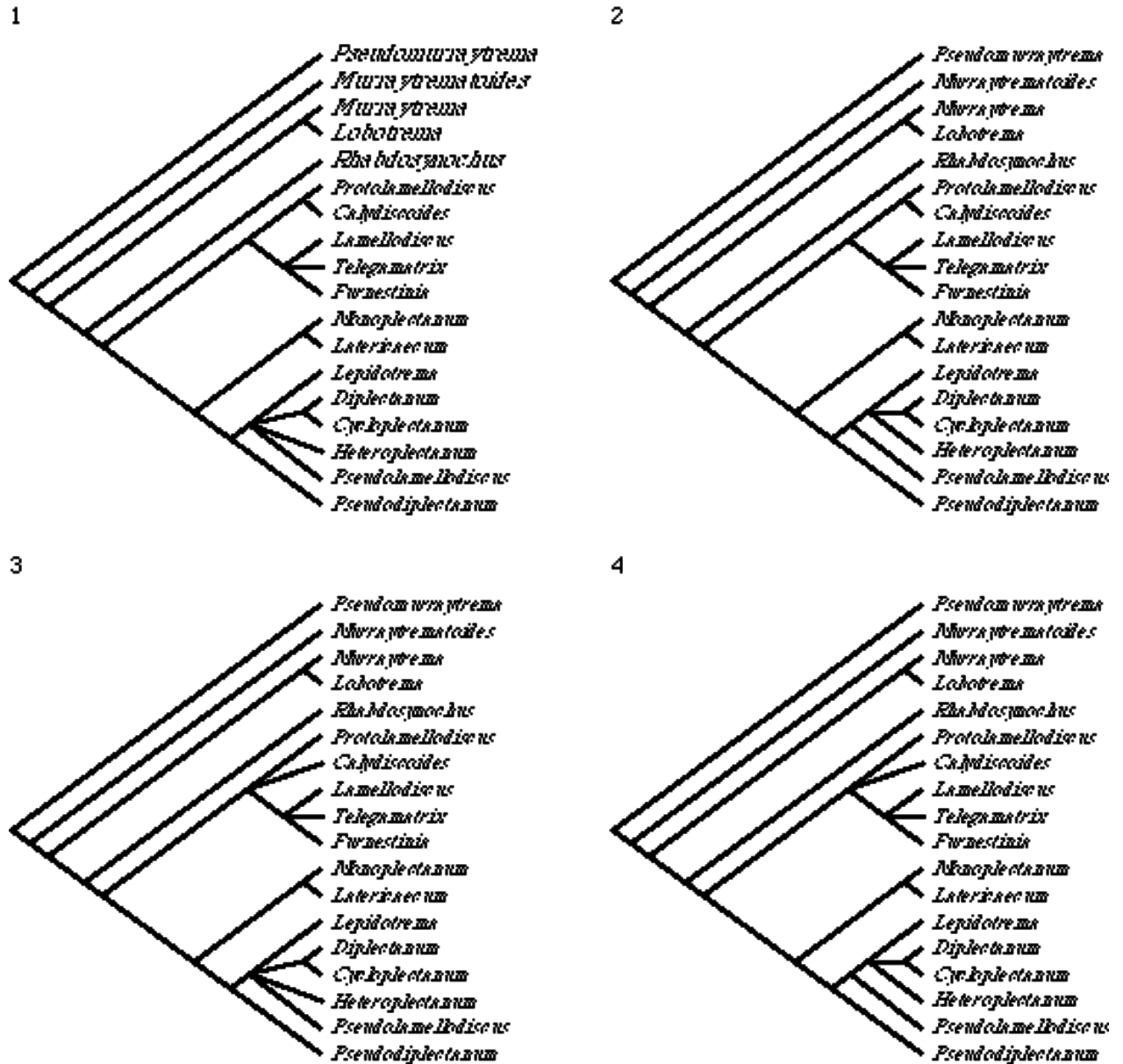
Figure IV.4: Arbres phylogénétiques des Diplectanidae obtenus par parcimonie après rep pondération des caractères.
