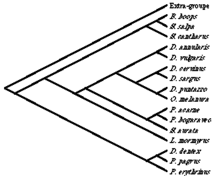
Figure IV.9 : Arbre phylogénétique des Sparidae obtenu par parcimonie à partir des séquences 16S + cyt-b.
